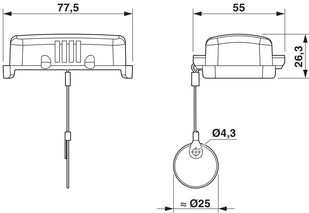
Maßzeichnung
