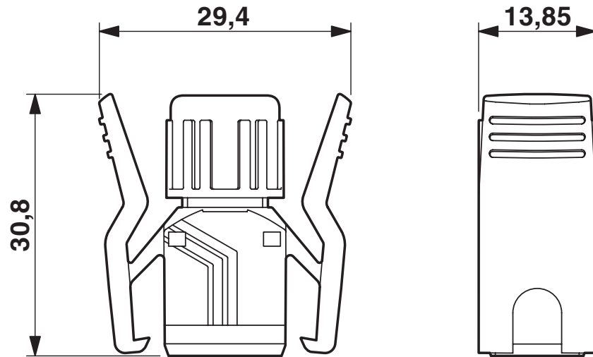
Dessin coté
