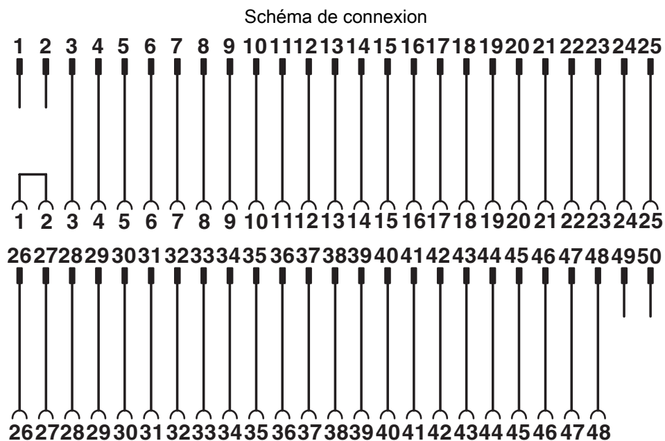
Schéma des connexions FLKM 50-PA-S400 (3-48)
