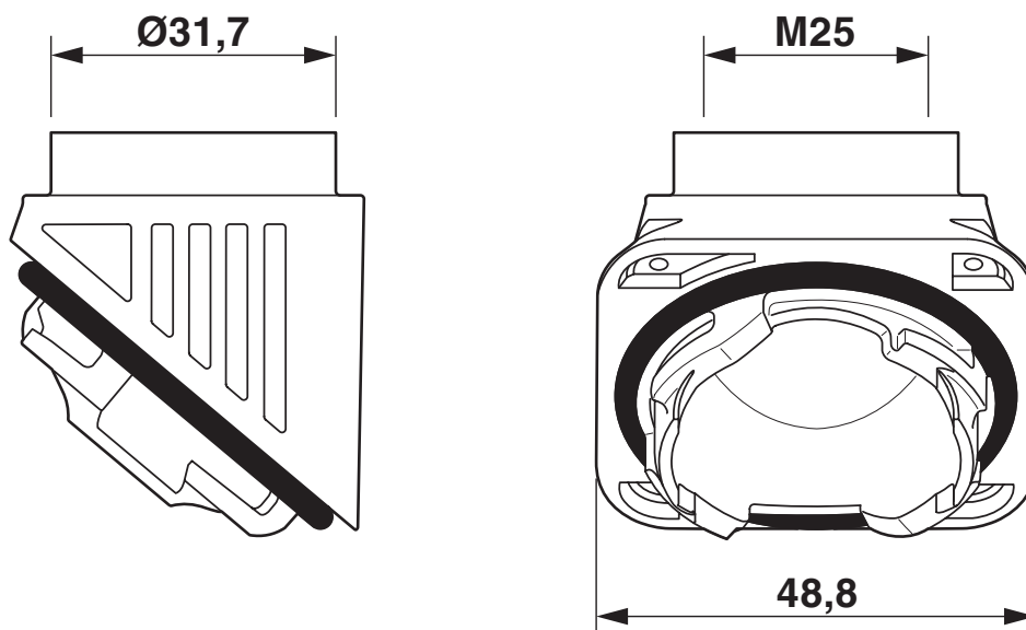
Maßzeichnung
