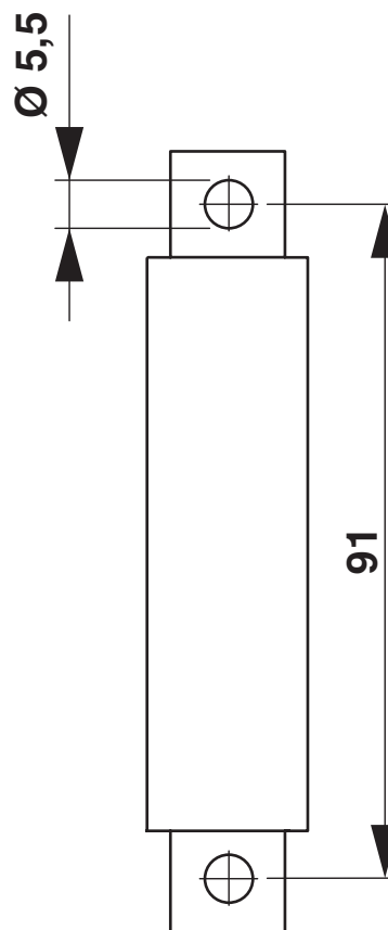
Dessin coté
