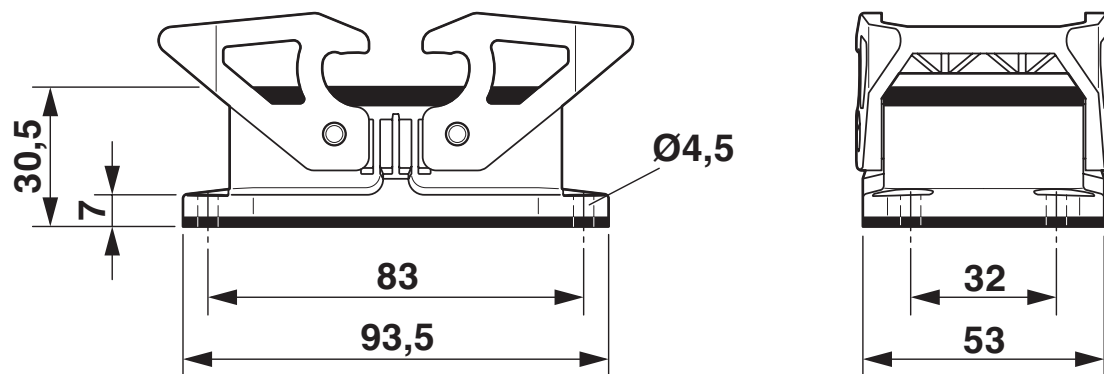
Dessin coté
