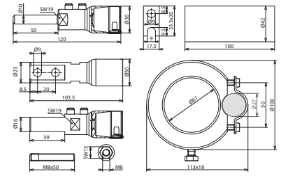
Maßbild HVI P LO ASS RAV KF 27 V2A
