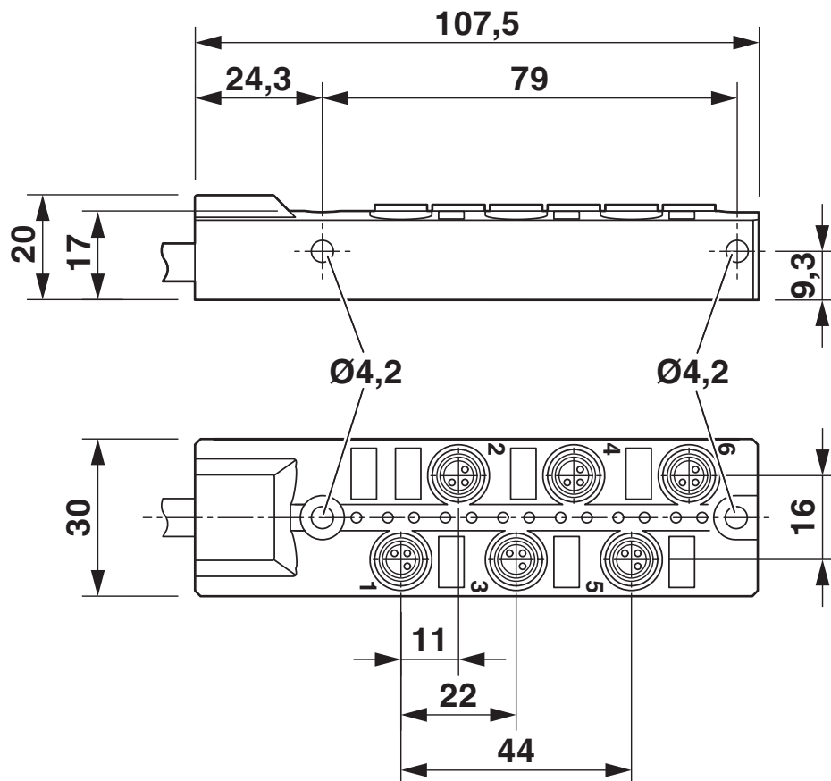
Dessin coté
