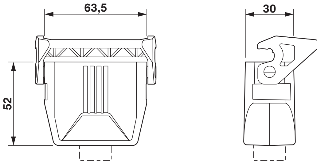
Maßzeichnung
