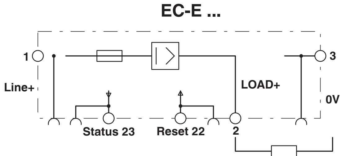
Diagrama eléctrico
