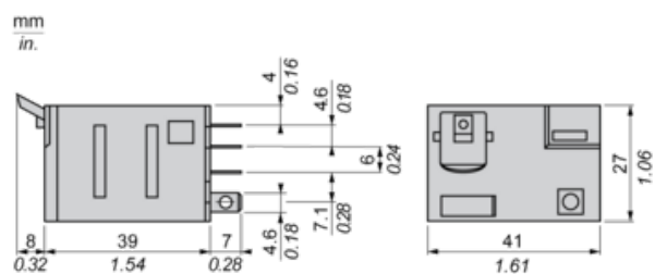
Vue côté broches
