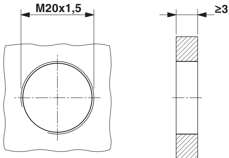
Maßzeichnung
