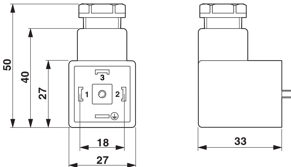
Dessin coté
