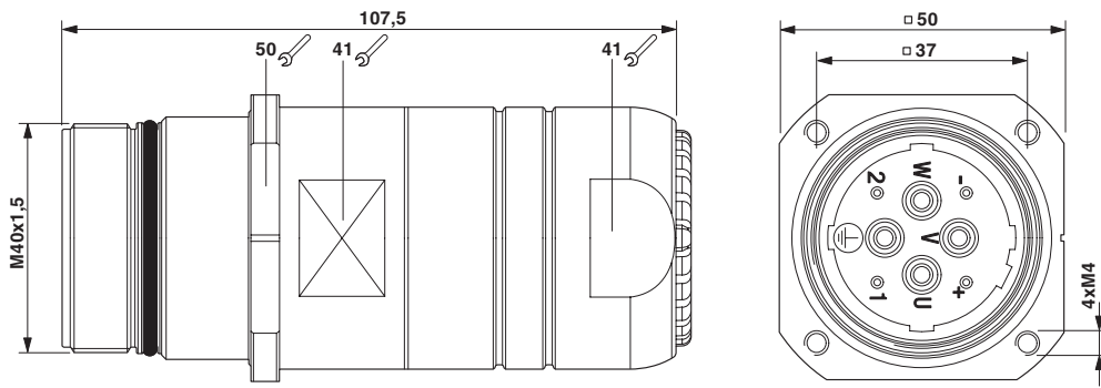
Dessin coté
