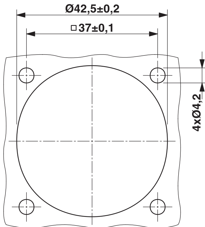
Dessin coté
