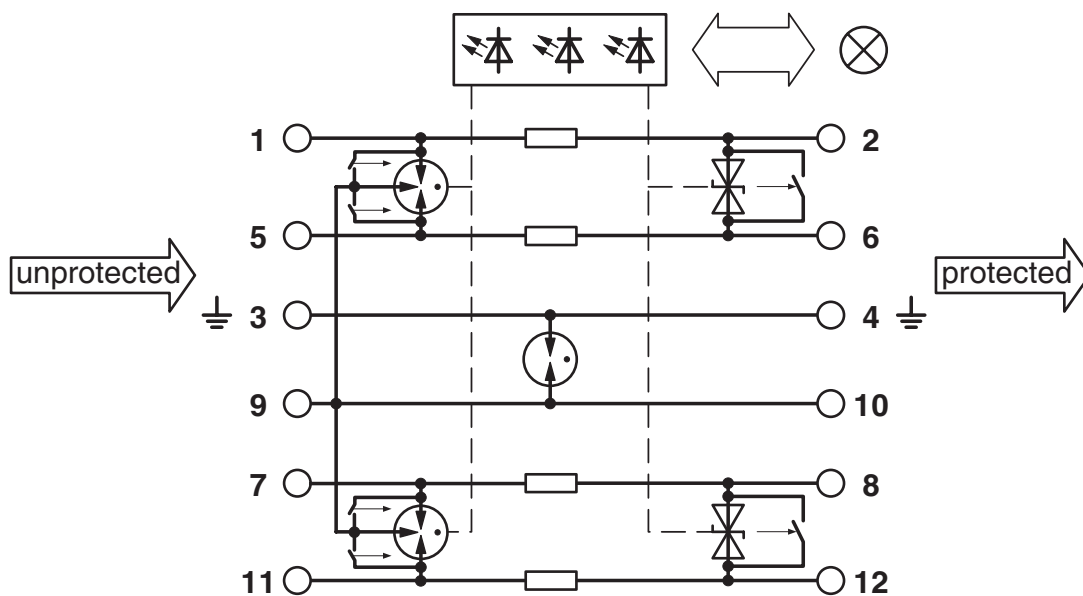
Diagrama eléctrico
