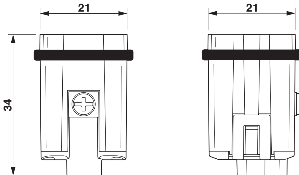
Maßzeichnung
