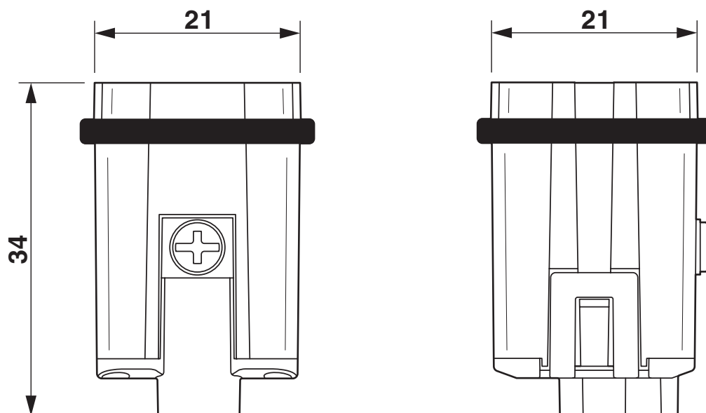
Dessin coté
