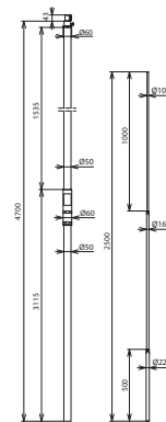
Maßbild SR D50 4700 FS22 2500 IP HVI GFK
