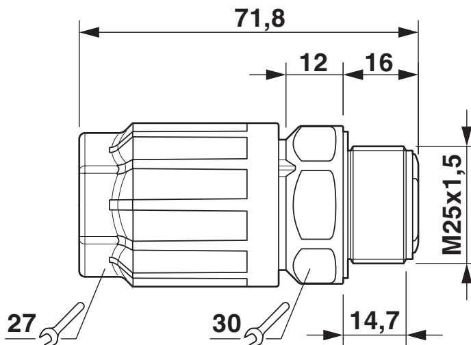
Maßzeichnung
