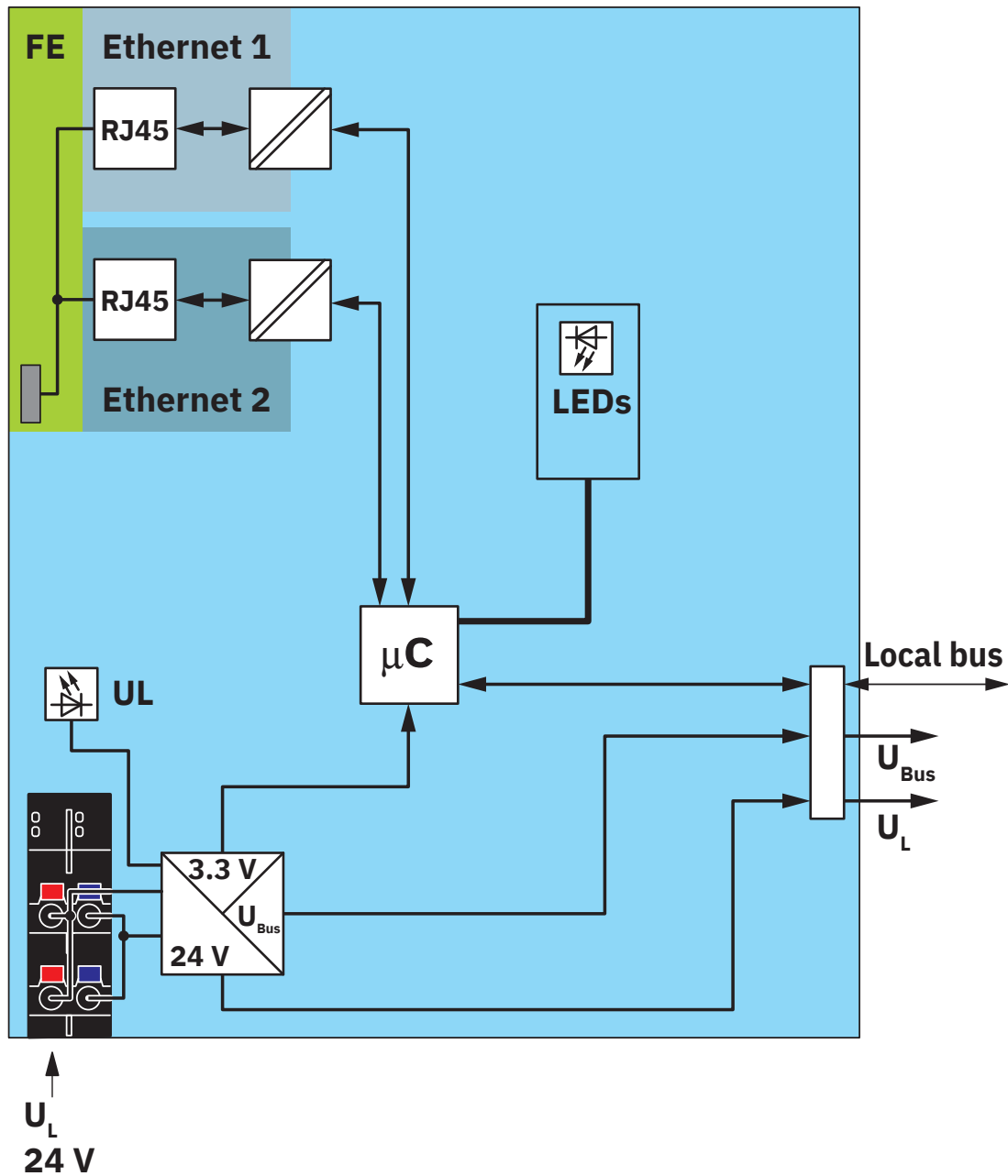
Blockschaltbild
