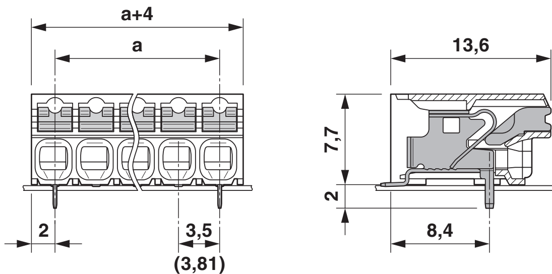
Maßzeichnung
