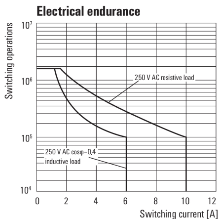
Elektrische Lebensdauer
