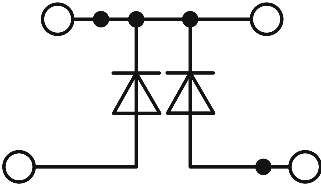
Schaltplan
