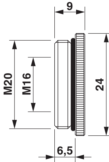
Maßzeichnung
