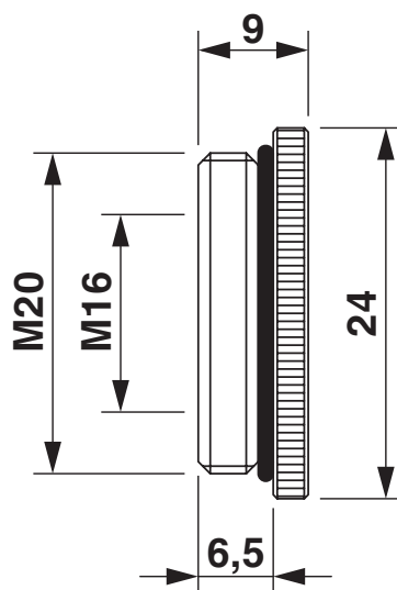
Esquema de dimensiones
