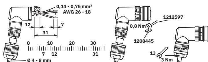
Funktionszeichnung
