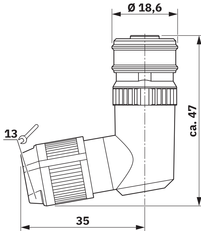
Maßzeichnung
