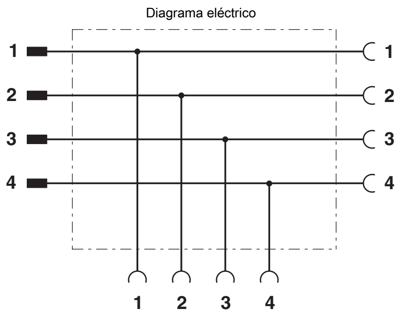
Ocupación de contactos del distribuidor T M12
