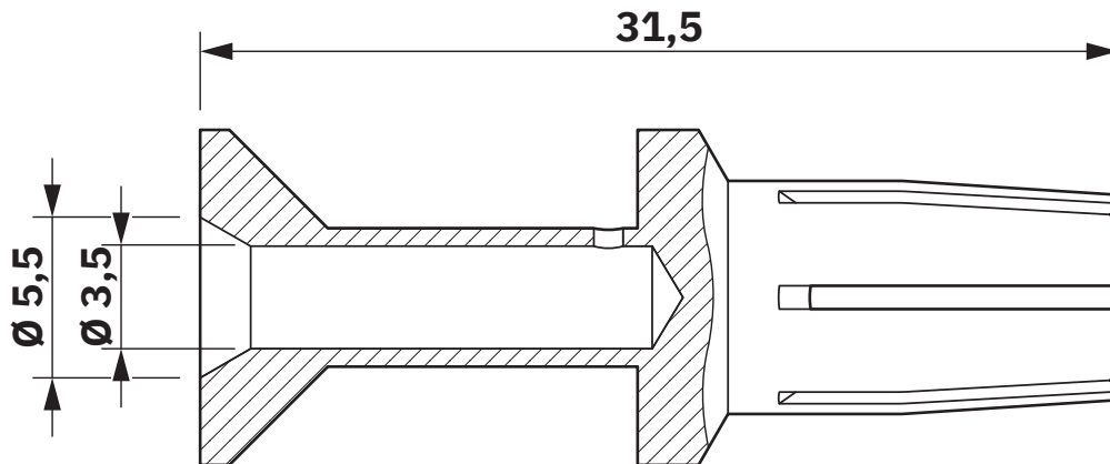
Maßzeichnung
