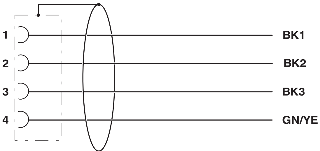
Schaltplan
