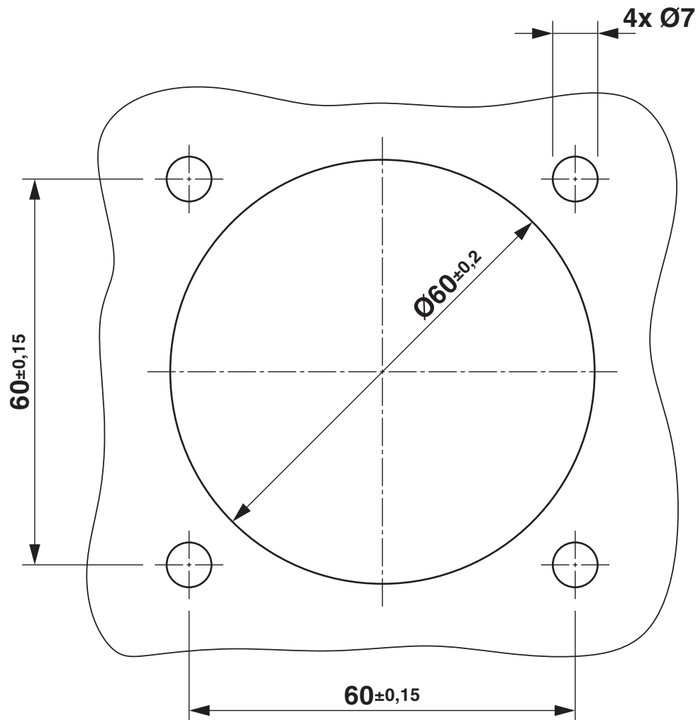
Bohrplan/Lötpadgeometrie
