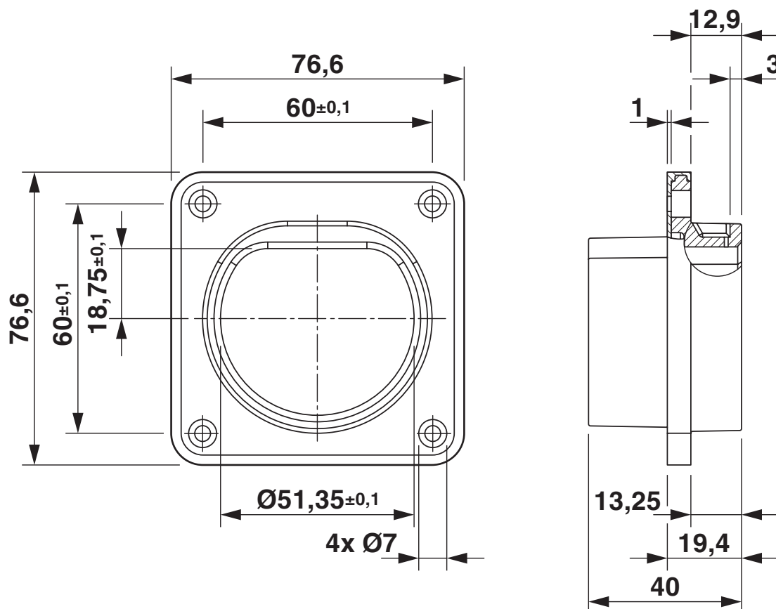
Dessin coté
