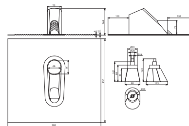
Maßbild DADS D10 16 48 AL SCH
