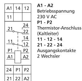
Anschlussbild
