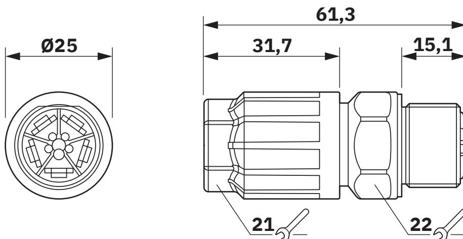
Maßzeichnung
