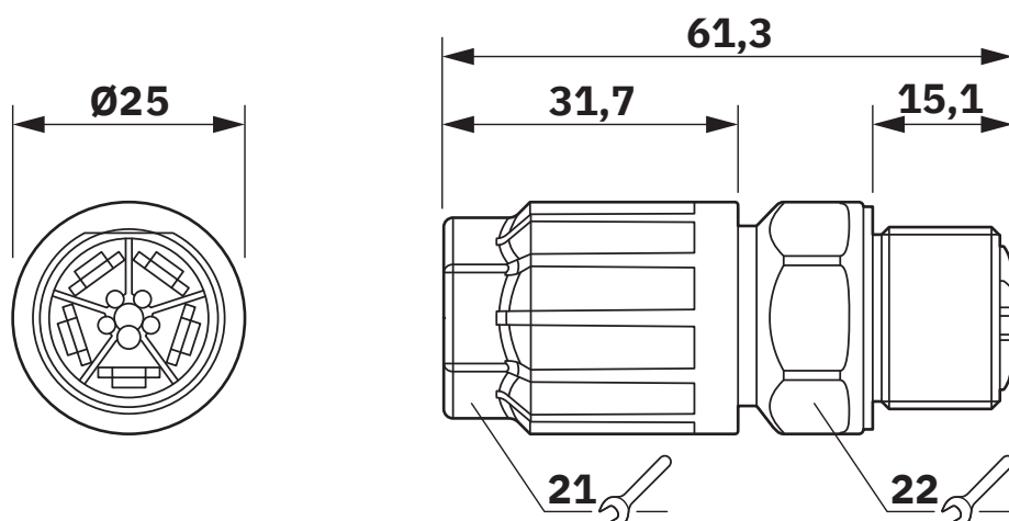
Dessin coté
