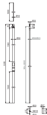
Maßbild HVI 20 M L6M SR3200 IP FSP1000
