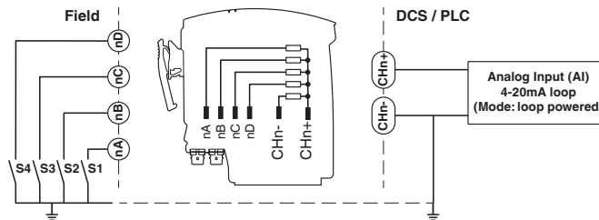
Plano esquemático
