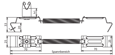
Maßbild DLH SG 8 H20 FG180.280 CU
