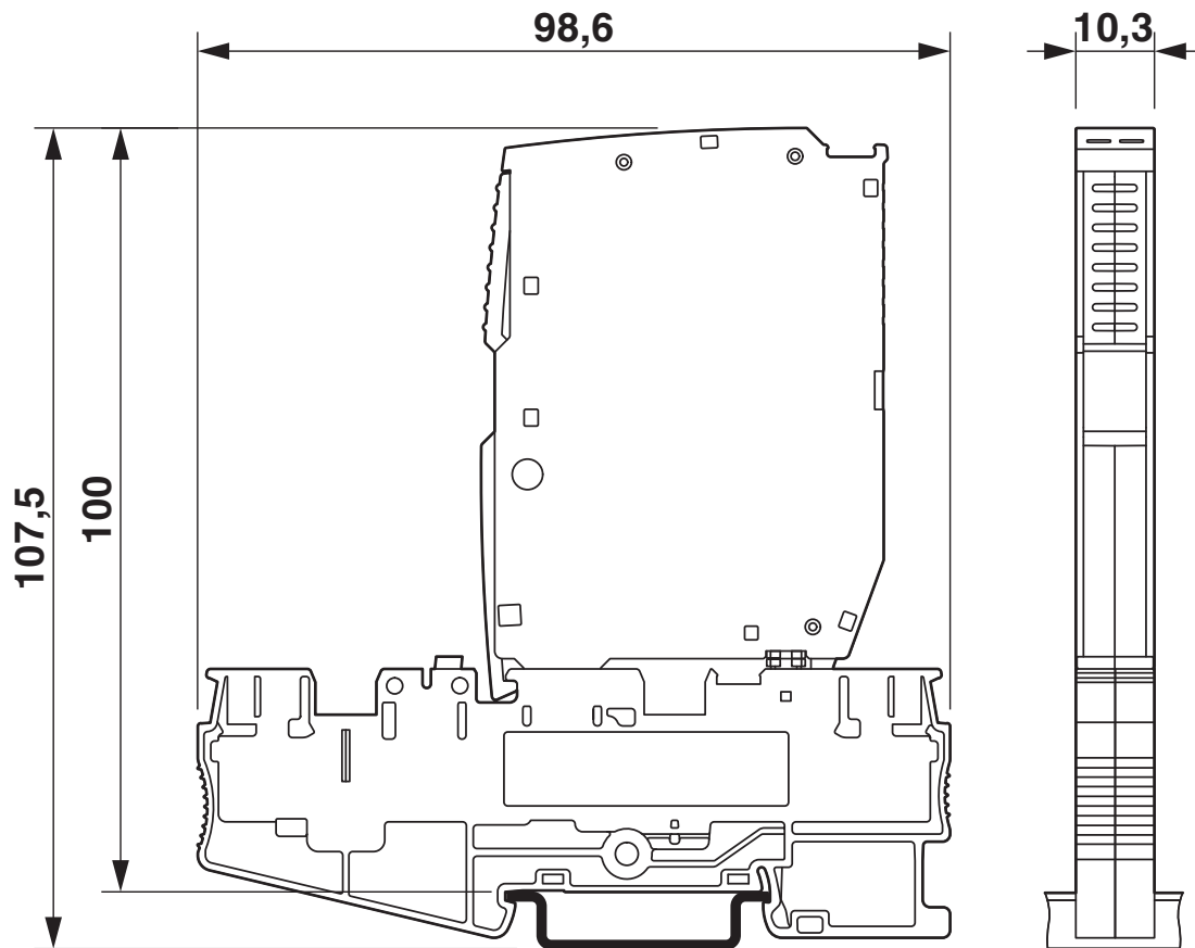
Dessin coté
