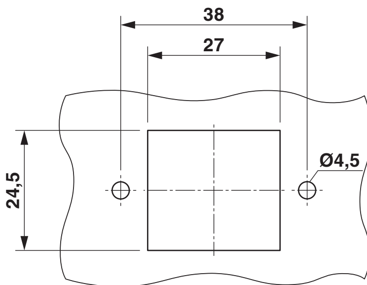
Dessin coté
