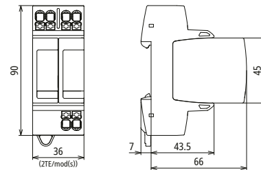
Maßbild DG MP TT 2P 275
