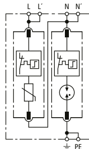
Prinzipialschaltbild DG MP TT 2P 275
