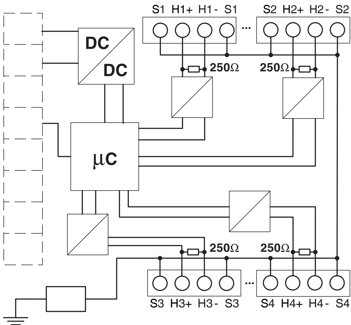
Schéma fonctionnel
