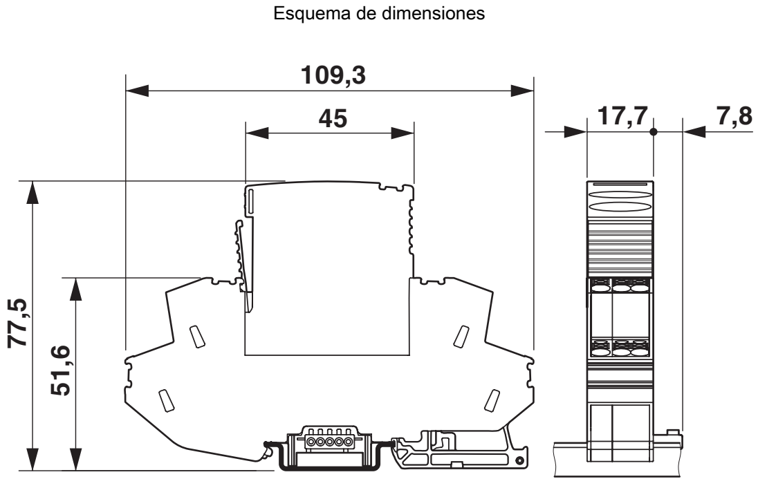
Plano esquemático
