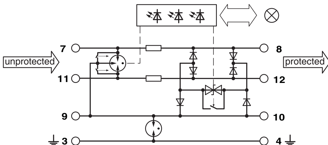
Diagrama eléctrico
