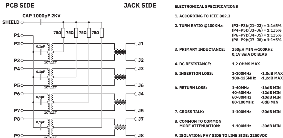
Diagrama eléctrico
