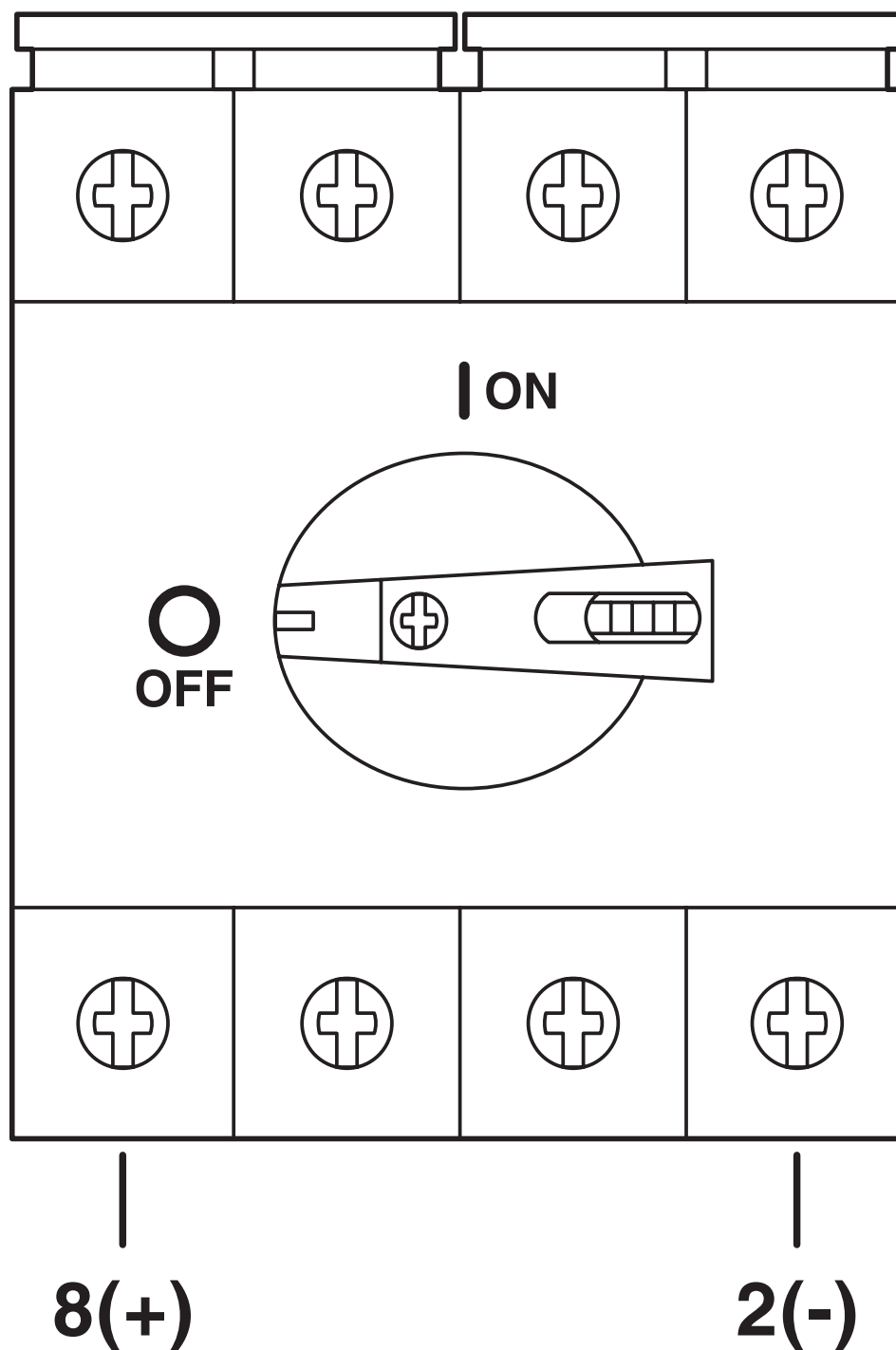
Dessin schématique
