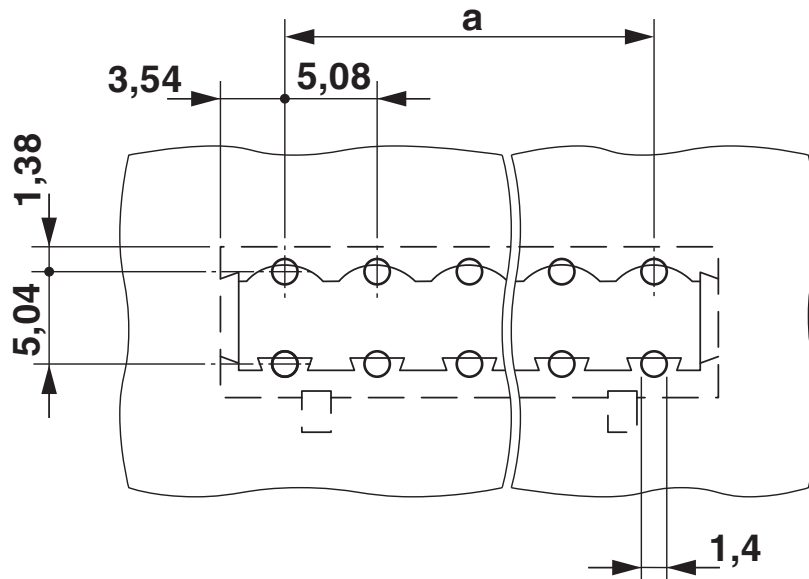
Bohrplan/Lötpadgeometrie
