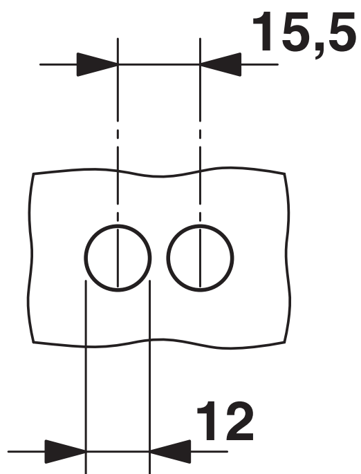
Dessin coté
