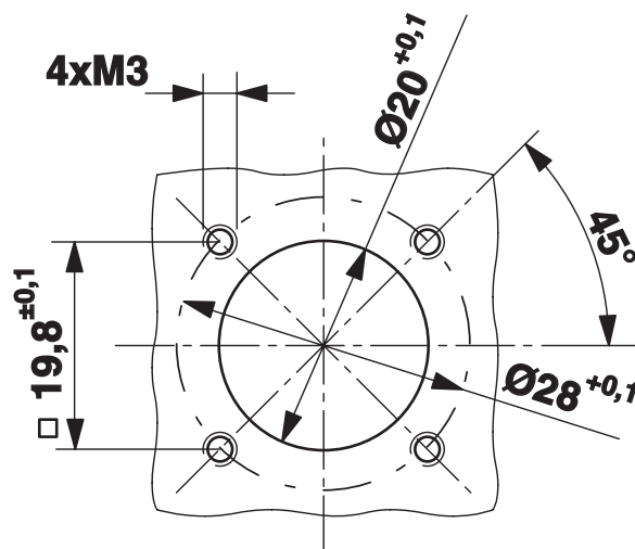
Schemazeichnung
