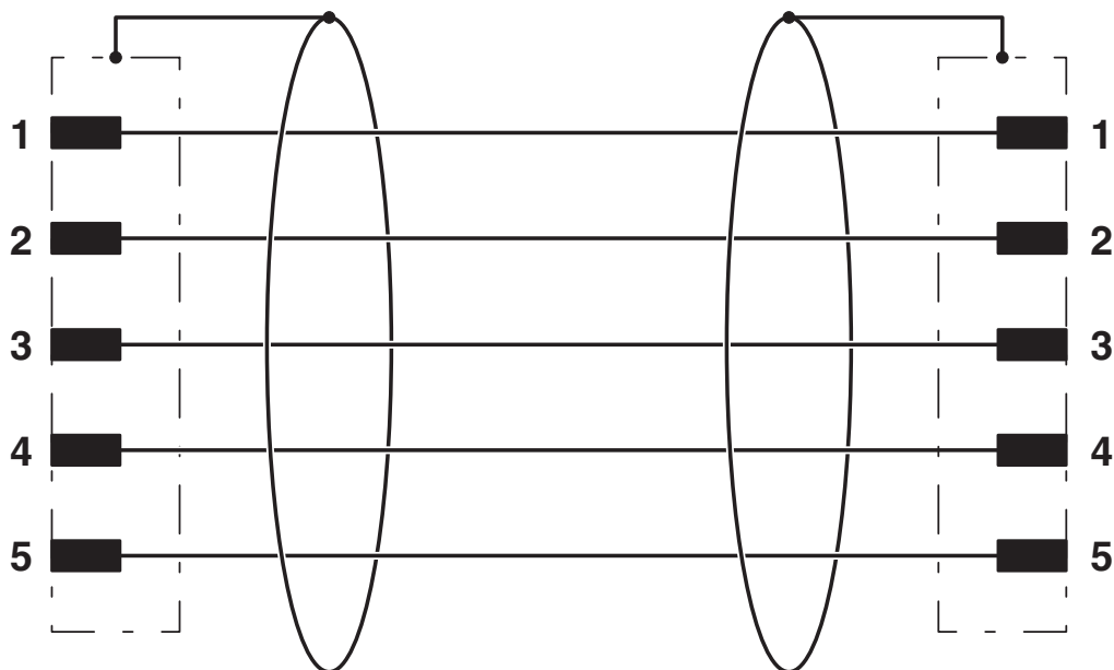
Schaltplan
