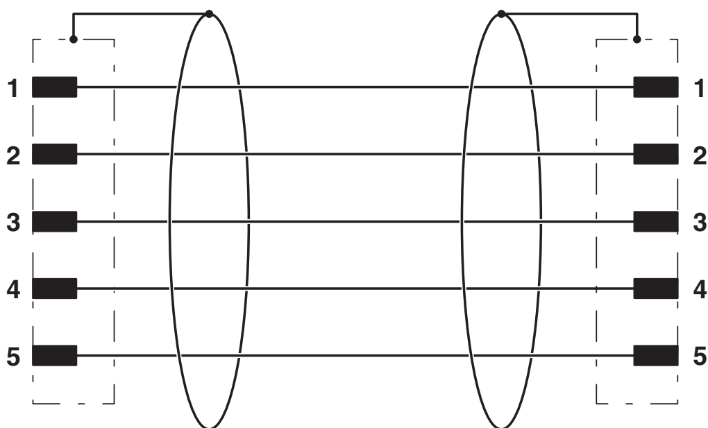
Diagrama eléctrico
